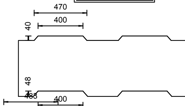
Coupe centrale
